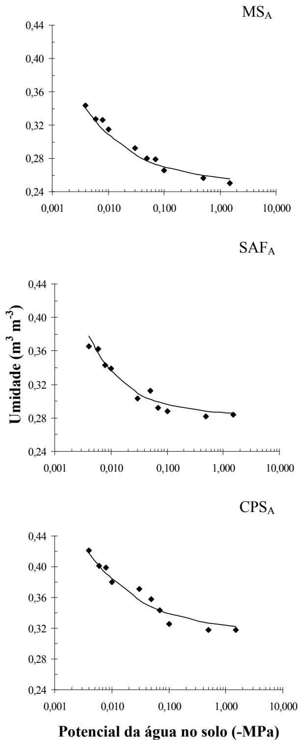
Figura 7 - Curva de retenção de água para os usos do solo avaliados em Araçá. Os pontos representam os dados observados e, a linha, a equação de ajuste conforme modelo de Van Genuchten. MS_A : mata secundária; SAF_A : sistema agroflorestal; CPS_A : cultivos a pleno sol.
