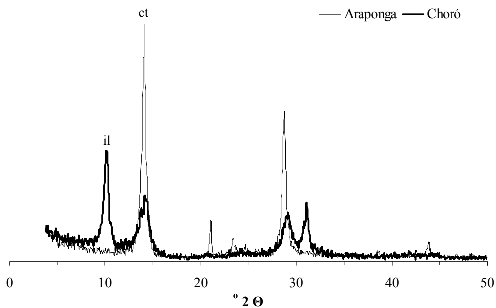
Figura 1 – Difratoograma de raios-X da fração argila dos solos estudados em Araponga (MG) e Choró (CE). il: ilita; ct: caulinita ( K_{\alpha} Co)
