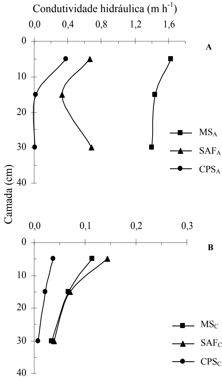
Figura 6– Valores médios de condutividade hidráulica do solo meio saturado ( m h^{-1} ) obtidos em laboratório para os sistemas avaliados em Araponga (A): MS A mata secundária, SAF A , sistema agroflorestal, CPS A cultivo a pleno sol; e Choró (B) MS C , mata secundária; SAF C , sistema agroflorestal; CPS C , consórcio a pleno sol.
